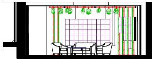
Coupe C-C
